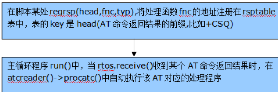
图5 regrsp() 流程图
