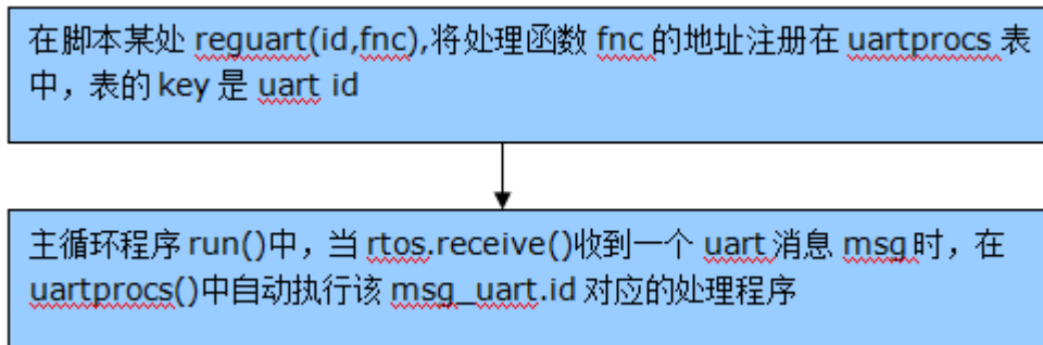
图6 reguart() 流程图
